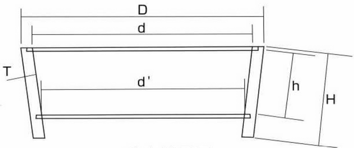
中央断面図
